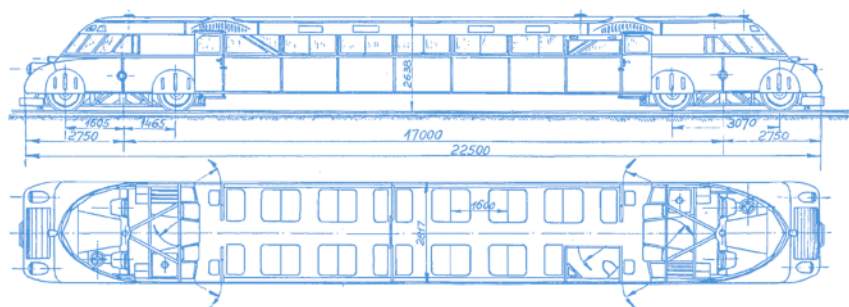
Wagon Diesel-hydr. (MAN-Austro-Daimler-Voith-Chrzanów), zbudowany przez Pierwszą Fabrykę Lokomotyw w Polsce.
